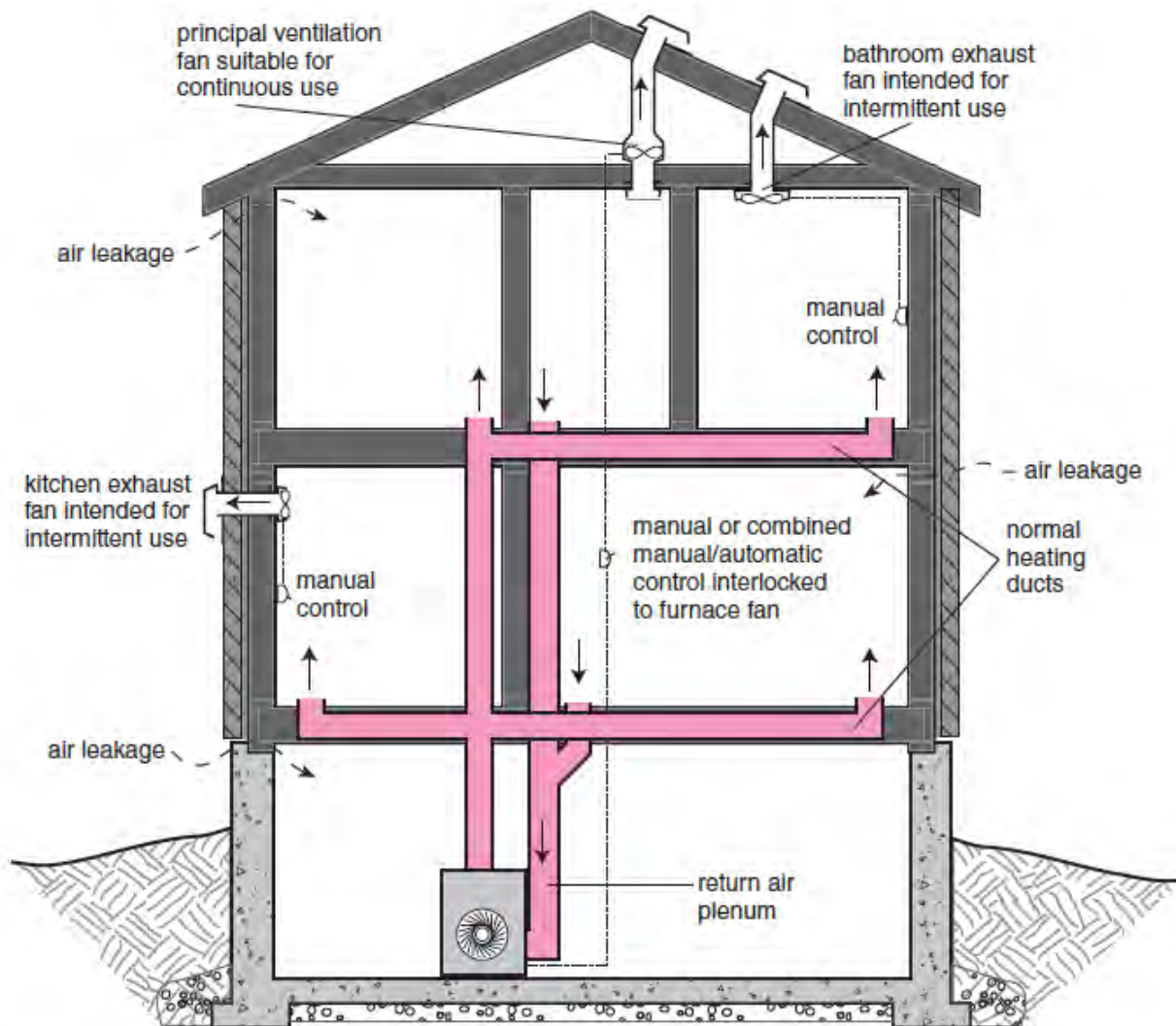
Figure A-9.32.3.6.
