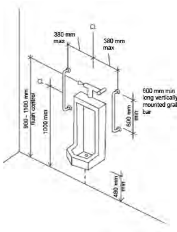
Figure A-3.8.3.10. Accessible Urinal
