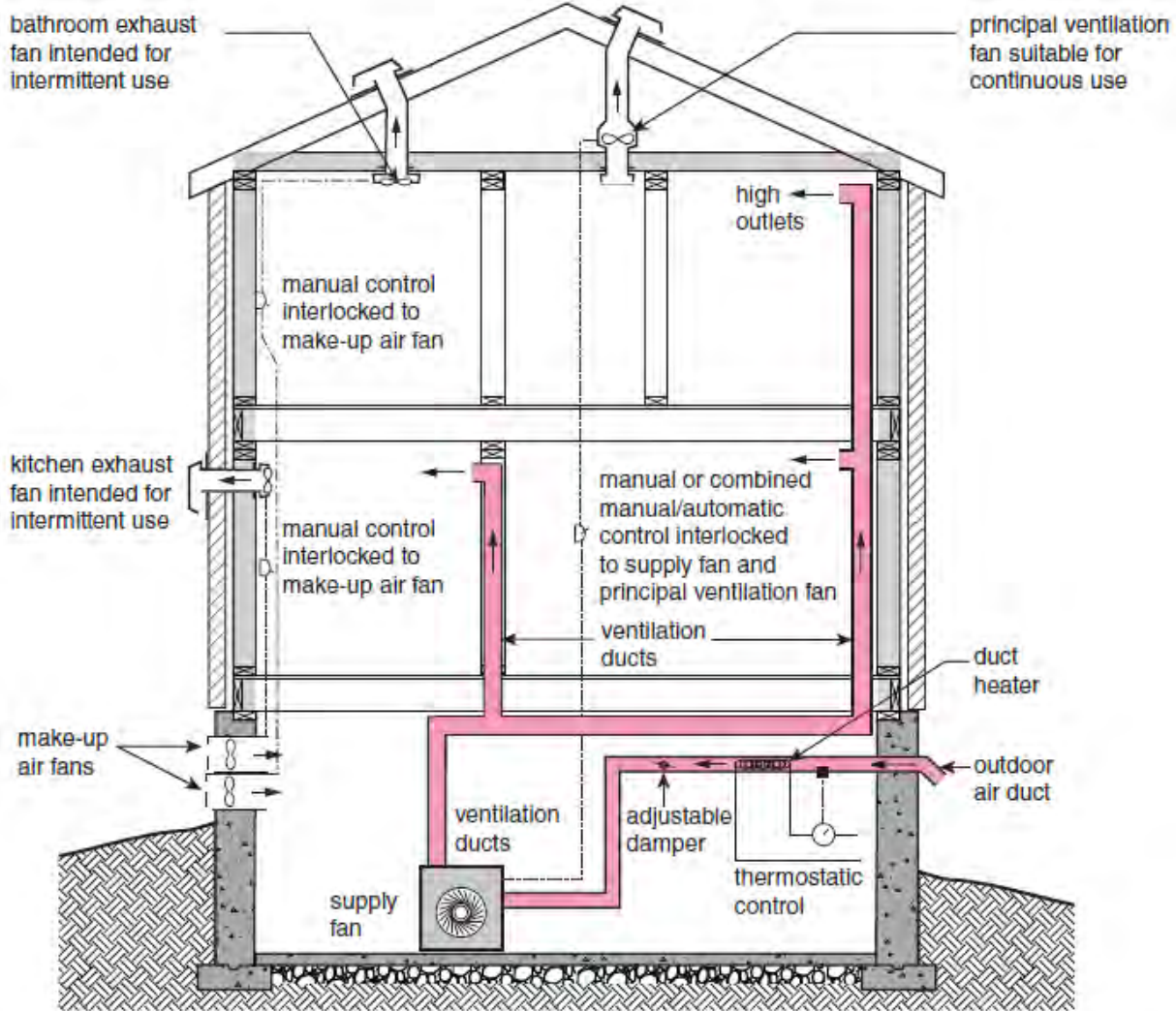
Figure A-9.32.3.3.-C
