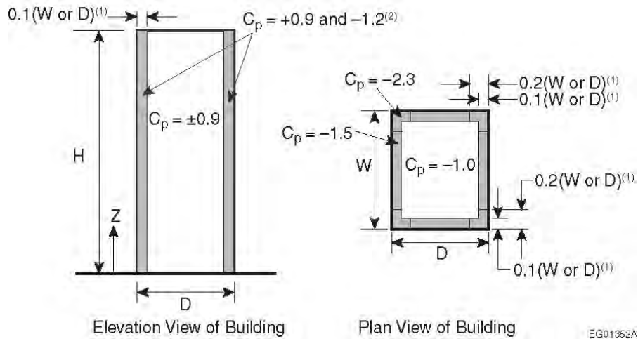
Figure A-4.1.7.5.(4)
